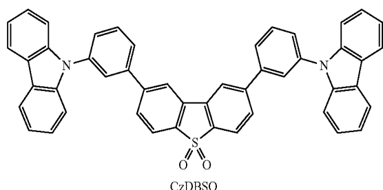
CzDBSO
